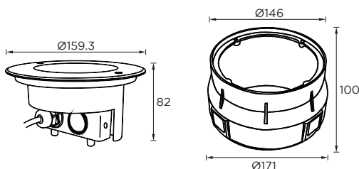
18W 3000K 10°
