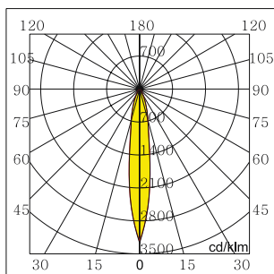
18W 3000K 10°
