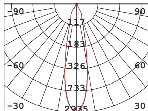
10W 3000K 36°
