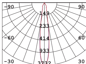
10W 3000K 24°
