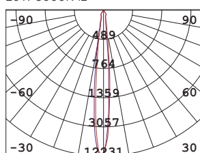
20W 3000K 24°
